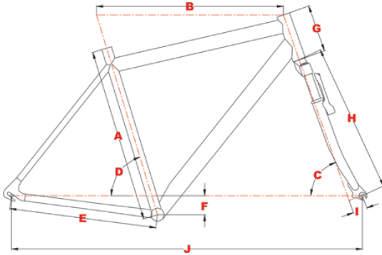
forma del telaio diamante
