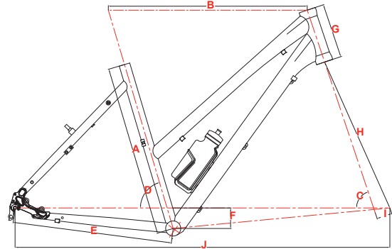
forma del telaio trapezio
